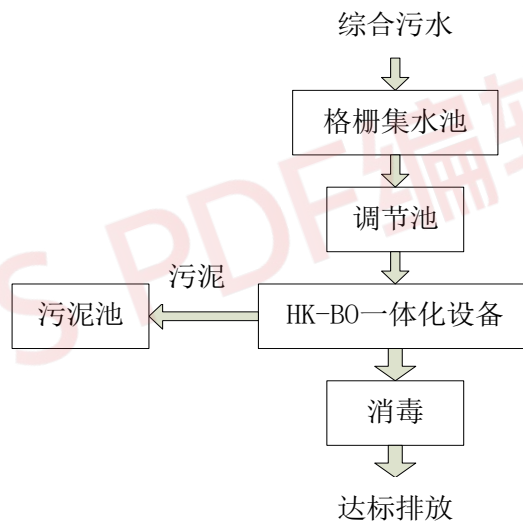
图 5-4 HK-BO 一体化污水处理设备工艺流程图
