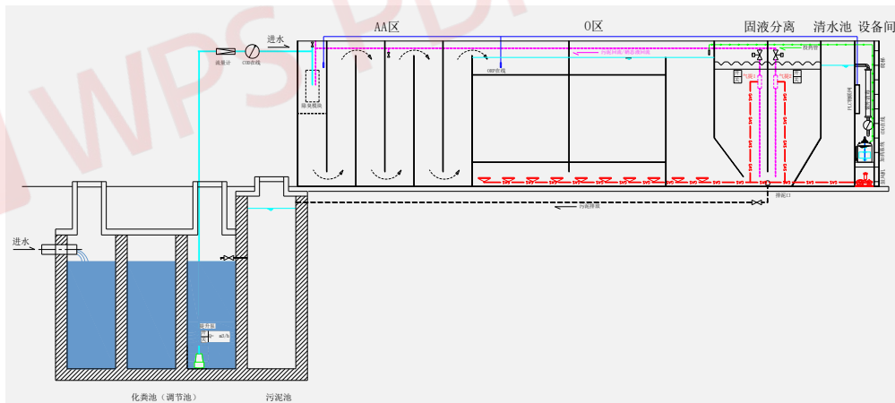
图 5-2“HIT”集装箱工艺流程图
