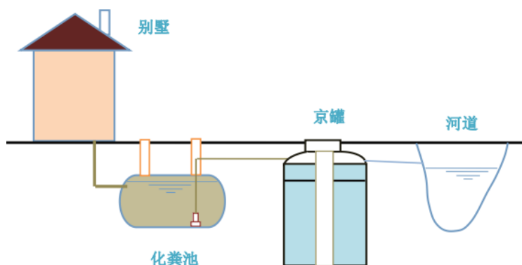
图 5-1 京罐工艺流程图
